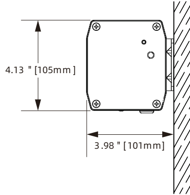
نصب دیواری
