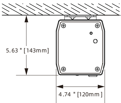
نصب سقفی
