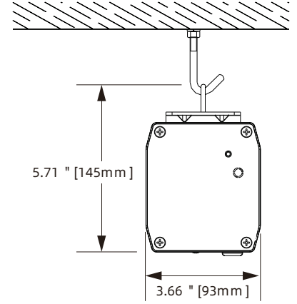
نصب معلق
