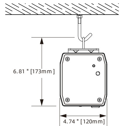
نصب معلق
